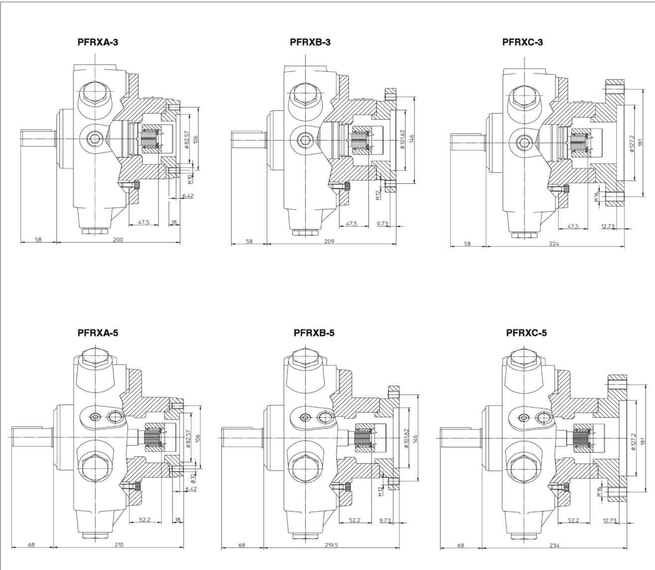
9 与叶片泵或齿轮泵联接时的尺寸 (mm)
